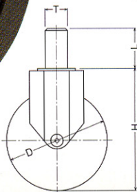
420EKR-R 100mm
